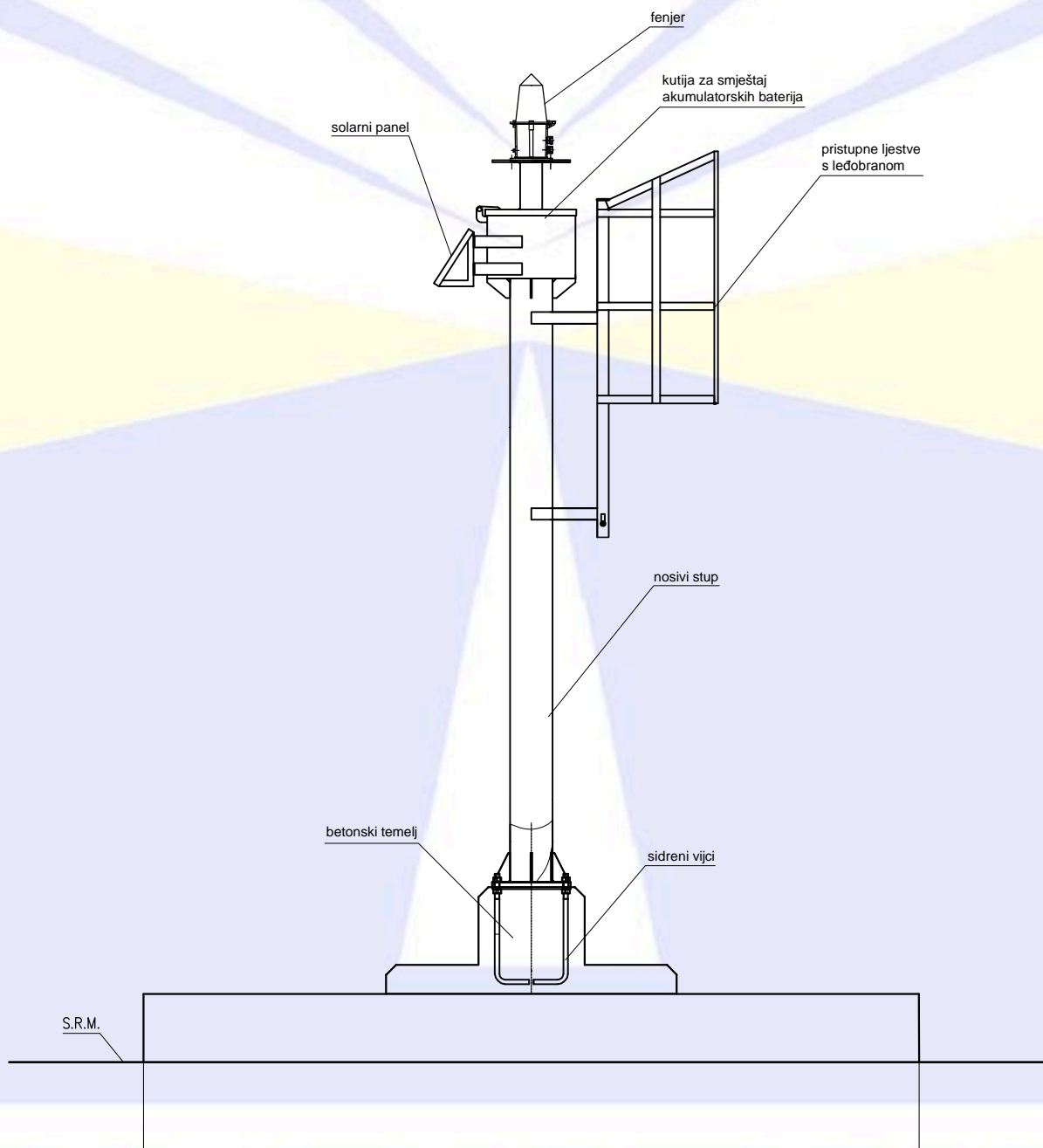
METALNI STUP - "PLOVPUT 2"
