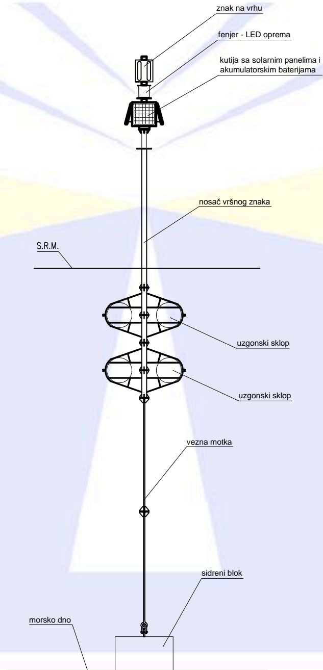
ZGLOBNO-ELASTIČNA OZNAKA - "PLOVPUT 2"
